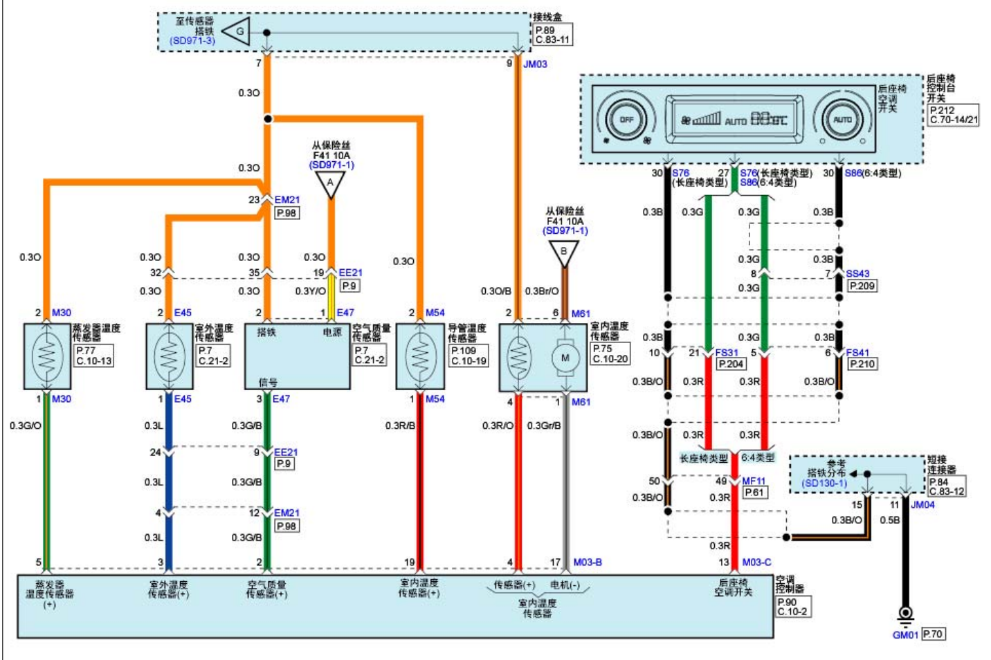
空调控制系统(自动)(4)
